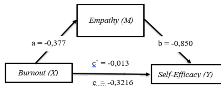
Gambar 2. Bagan bentuk mediasi sederhana
