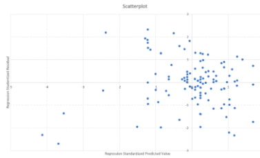
Gambar 1. Scatterplot Uji Heteroskedastisitas
